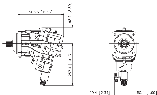
Regolatore RPS RPS Control
